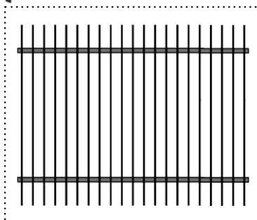
VUE DE FACE DE LA GRILLE
