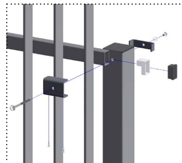
SYSTÈME DE FIXATION ROBUSTE
